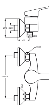
B 9382 AA Baterie sprchová nástěnná páková
