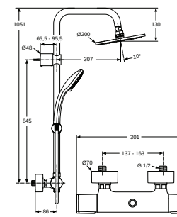
A5923AA Sprchový set s termostatickou baterií a hlavovou i ruční sprchou
