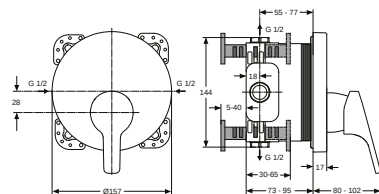
A5902AA Sprchová podmítková páková baterie (nadomítková část)
