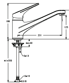
B0124AA Dřezová stojánková páková baterie, výtok 231 mm
