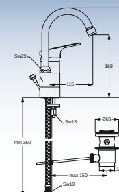
B 9380 AA Baterie umyvadlová stojánková páková
