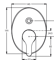
B 9390 AA Podomítková vanová páková baterie
