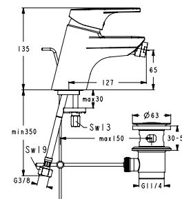
B0099AA Bidetová stojánková páková baterie, výtok 127 mm
