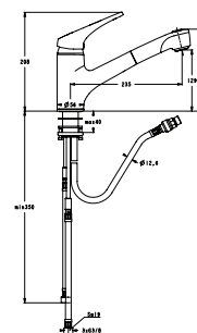
B0128AA Dřezová stojánková páková baterie s vytahovací sprškou, výtok 235 mm
