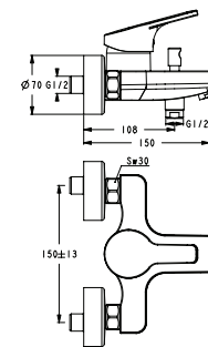
B0102AA Vanová nástěnná páková baterie bez příslušenství, výtok 150 mm
