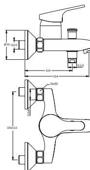
B 9383 AA Baterie vanová nástěnná páková
