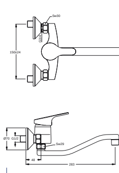
B 9385 AA Baterie dřezová nástěnná páková
