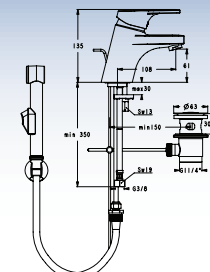
B0097AA Umyvadlová stojánková páková baterie s ruční sprškou, výtok 108 mm
