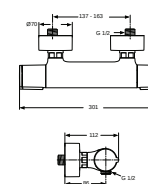
A5916AA Sprchová nástěnná termostatická baterie
