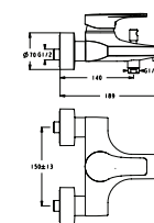
B0122AA Vanová nástěnná páková baterie, výtok 189 mm
