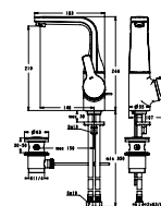
B0114AA; B0115AA Umyvadlová stojánková páková baterie, výtok 140 mm
