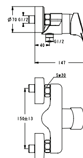
B0100AA Sprchová nástěnná páková baterie
