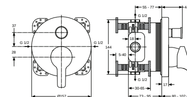
A5903AA; A5904AA Vanová podmínková páková baterie s přepínačem (nadomítková část)
