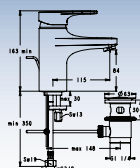
B0109AA; B0110AA Umyvadlová stojánková páková baterie s výpustí, výtok 115 mm B0111AA – bez výpustí, výtok 115 mm
