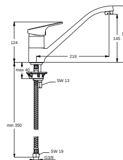
B 9384 AA Baterie dřezová stojánková páková
