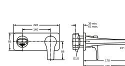
A5909AA – výtok 178 mm A5910AA – výtok 222 mm Umyvadlová podomítková páková baterie (nadomítková část)
