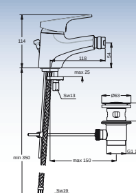
B 9381 AA Baterie bidetová stojánková páková s výpustí
