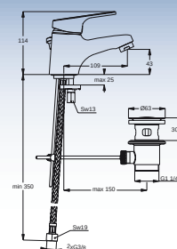
B 9378 AA s výpustí B 9376 AA bez výpustě Baterie umyvadlová stojánková páková
