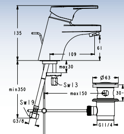
B0091AA; B0092AA; B0093AA; B0094AA; B0095AA Umyvadlová stojánková páková baterie s výpustí, výtok 109 mm
