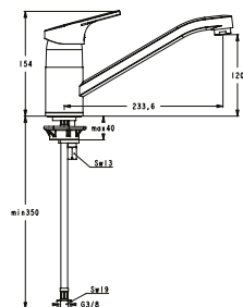
B0104AA Dřezová stojánková páková baterie, výtok 234 mm
