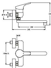
B0104AA – výtok 234 mm B0106AA – výtok 200 mm Baterie bidetová
