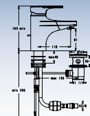
B0113AA Umyvadlová stojánková páková baterie se sprškou, výtok 118 mm
