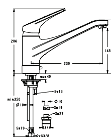
B0126AA Dřezová stojánková páková baterie, výtok 230 mm (s ventilem pro pračku, myčku)
