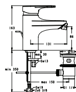
B0119AA Bidetová stojánková páková baterie, výtok 131 mm
